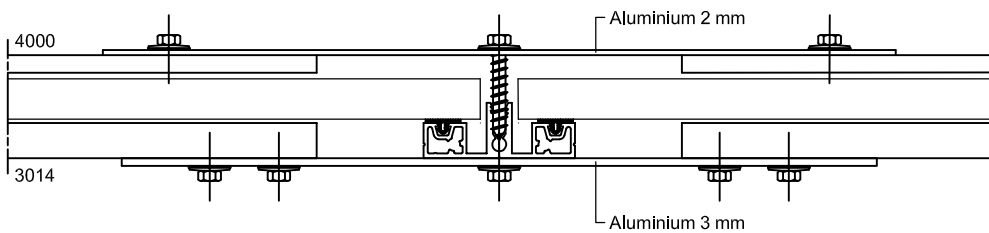
Doorsnede A - A
